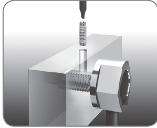
고정나사 설치
